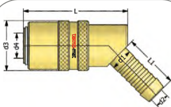
Standard hose tail socket 45° Kupplung mit 45° Standard-Schlauchtülle
