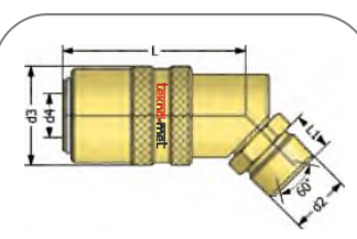
Cylindrical Male Thread socket 45° Kupplung mit 45° Aussengewinde zylindrisch
