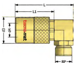
Cylindrical Thread socket 90° Kupplung mit 90° Aussengewinde zylindrisch BSP
