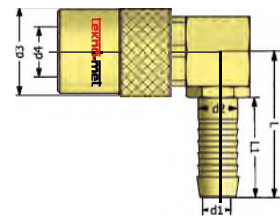
Standard hose tail socket 90° Kupplung mit 90° Standard-Schlauchtülle
