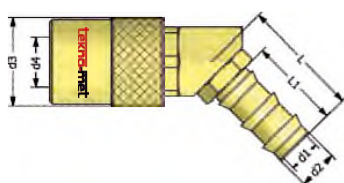
Push-Lock hose tail socket 45° Kupplung mit 45° Schnellsteck-Schlauchtülle
