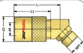
NPT Thread socket 45° Kupplung mit 45° Aussengewinde NPT
