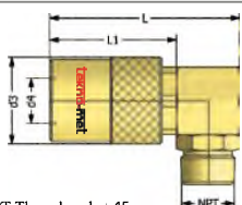
NPT Thread socket 45° Kupplung mit 45° Aussengewinde NPT
